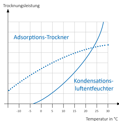
Leistungscharakteristik
