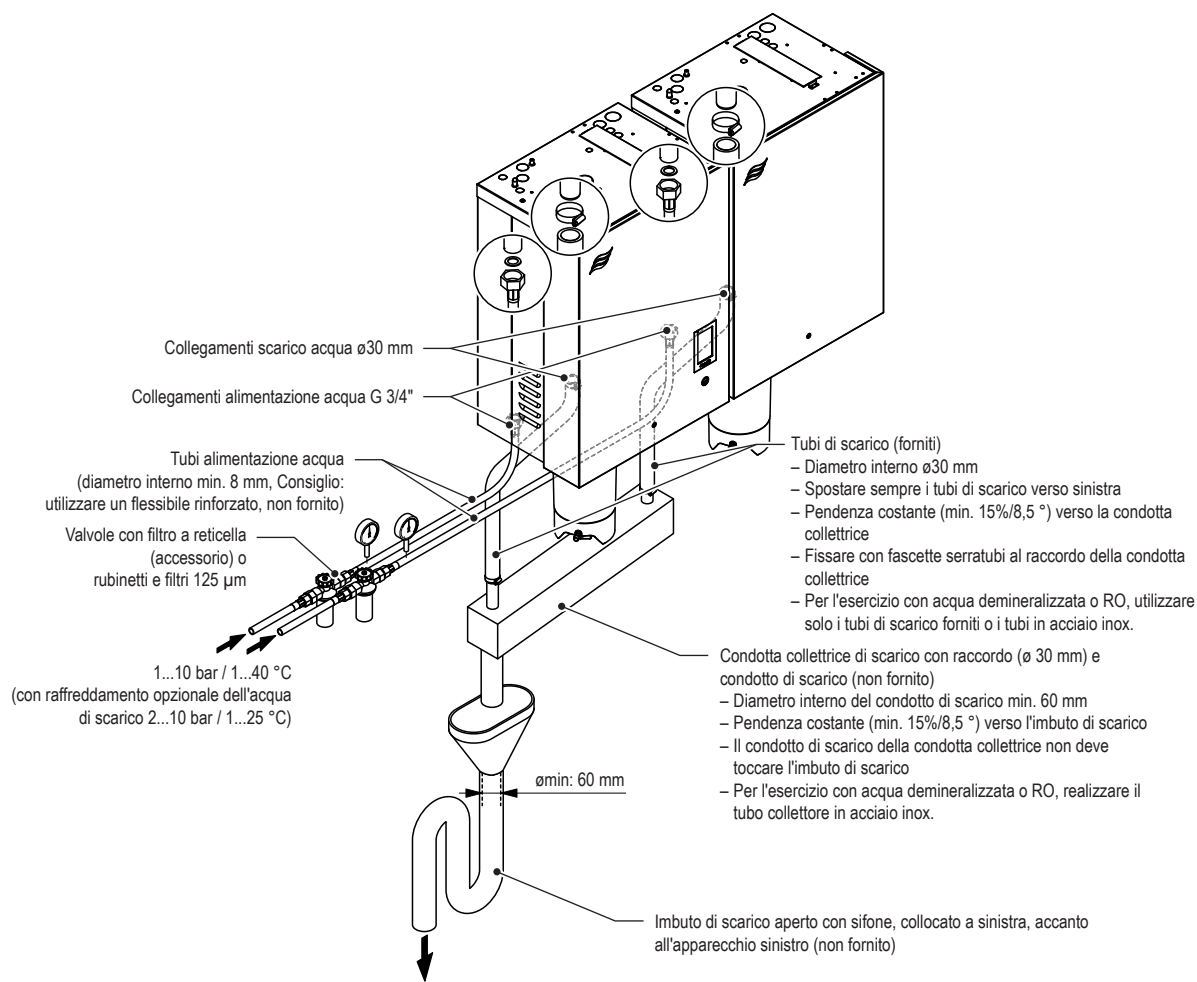
Fig. 24: Panoramica dell'installazione idraulica per i dispositivi doppi "M"
