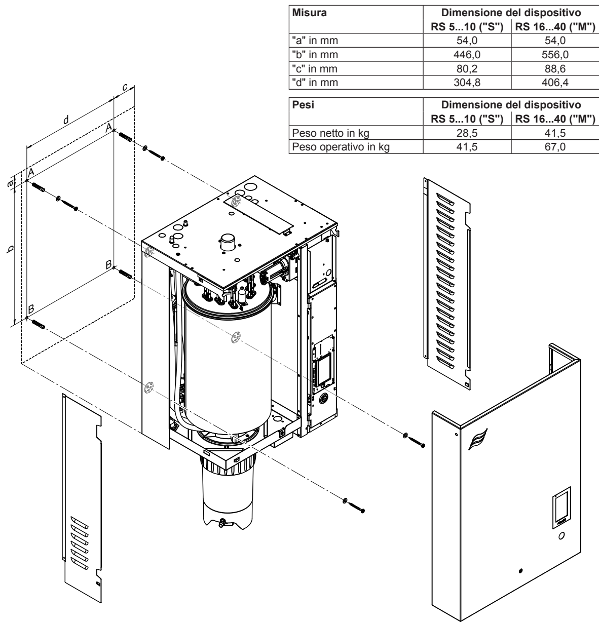
Fig. 11: Schema del montaggio standard dei moduli singoli piccolo e medio
