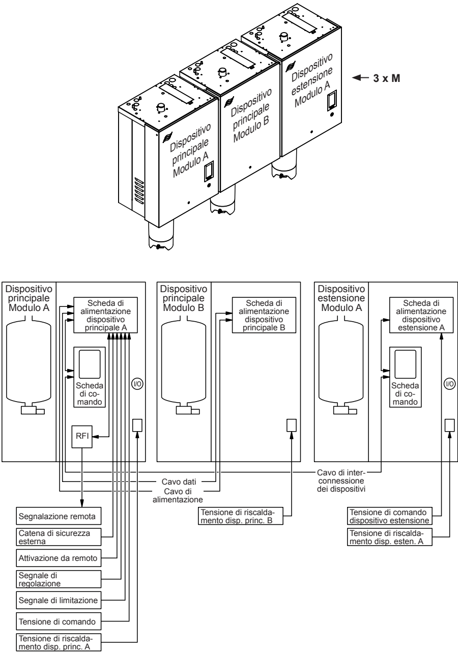
Fig. 4: Panoramica sistemi interconnessi (3 x "M")
