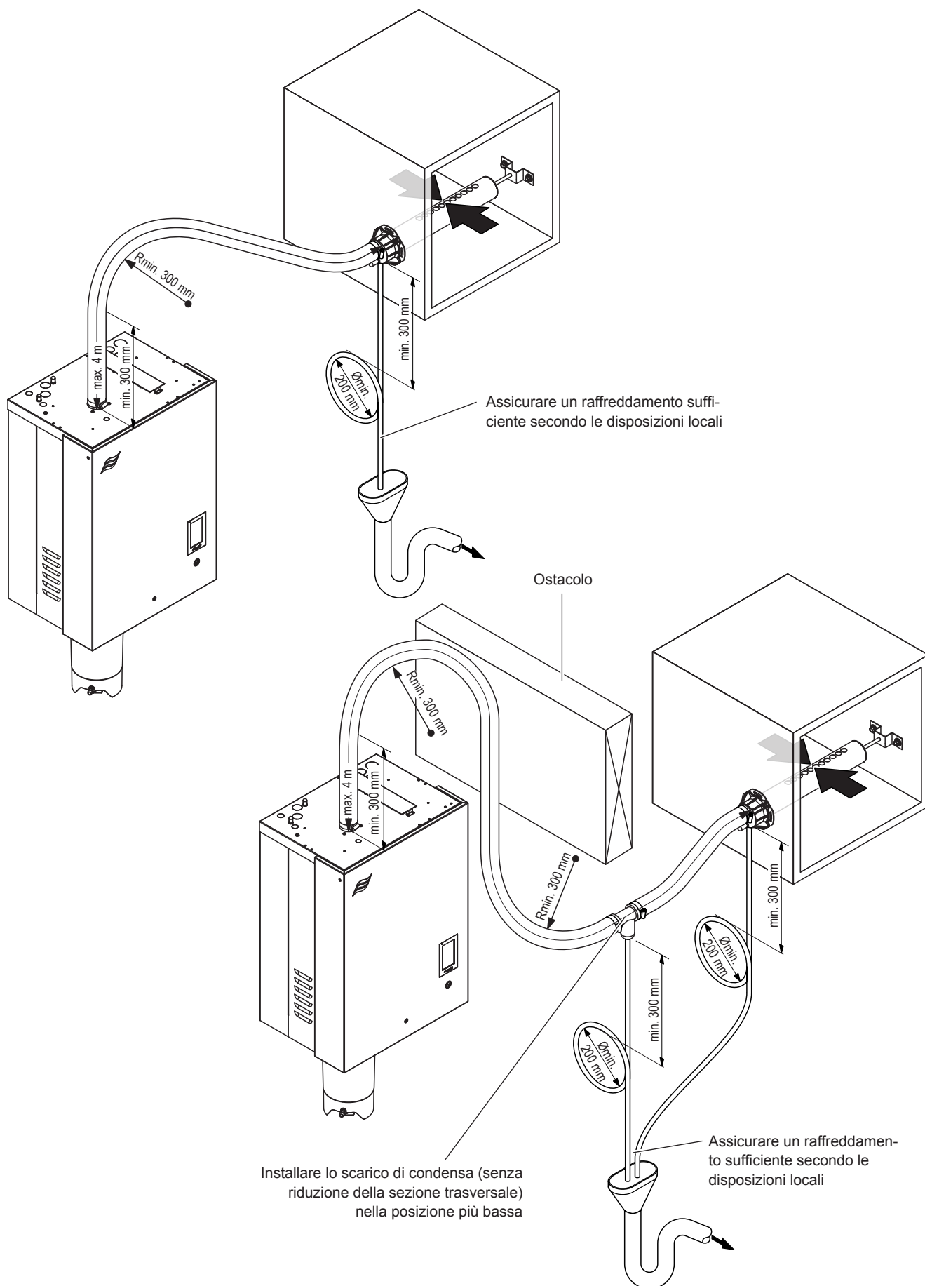
Fig. 19: Il distributore di vapore è montato a meno di 500 mm sopra o sotto l'angolo superiore dell'apparecchio
