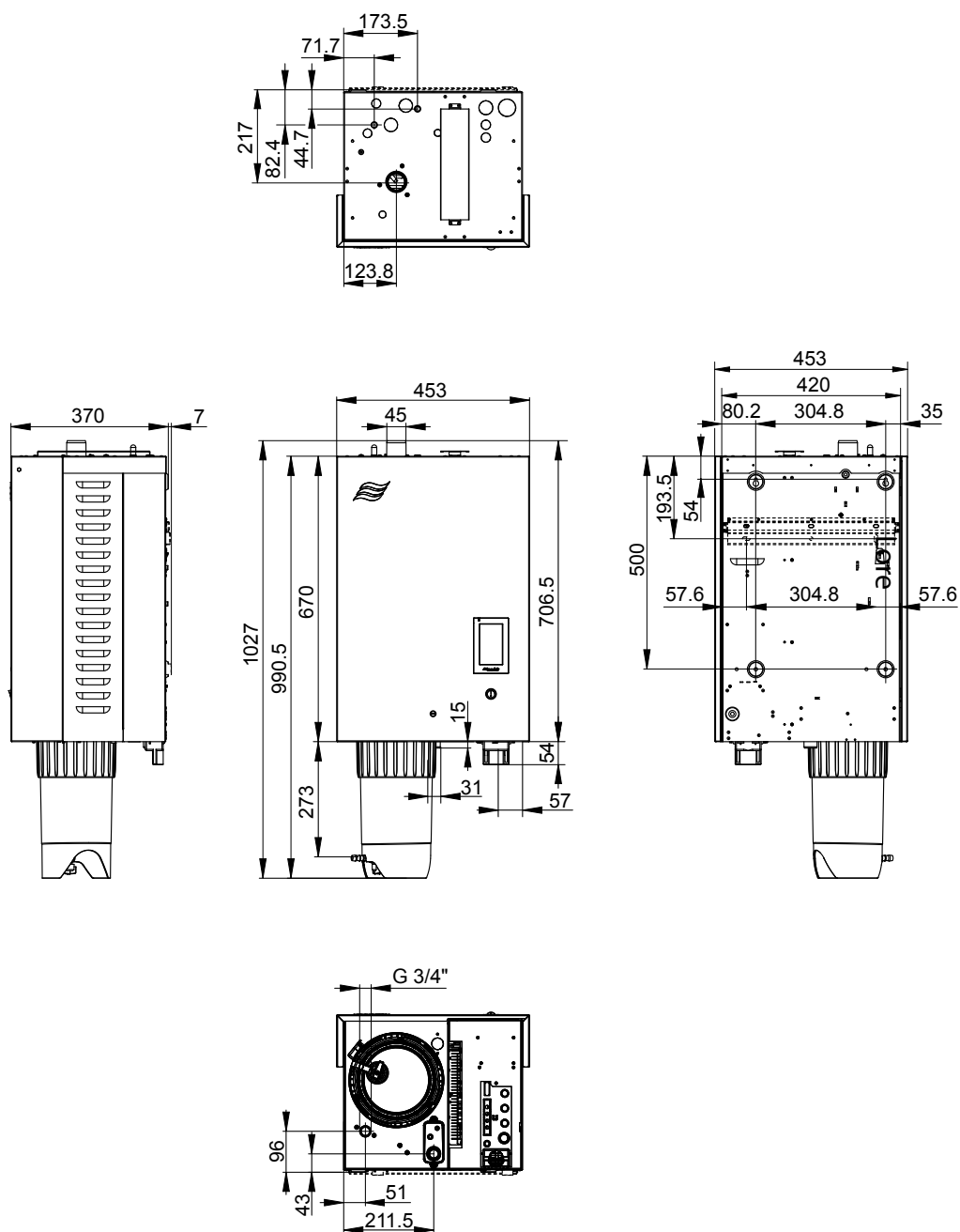
Fig. 34: Dimensioni del modulo "S" (misure in mm)
