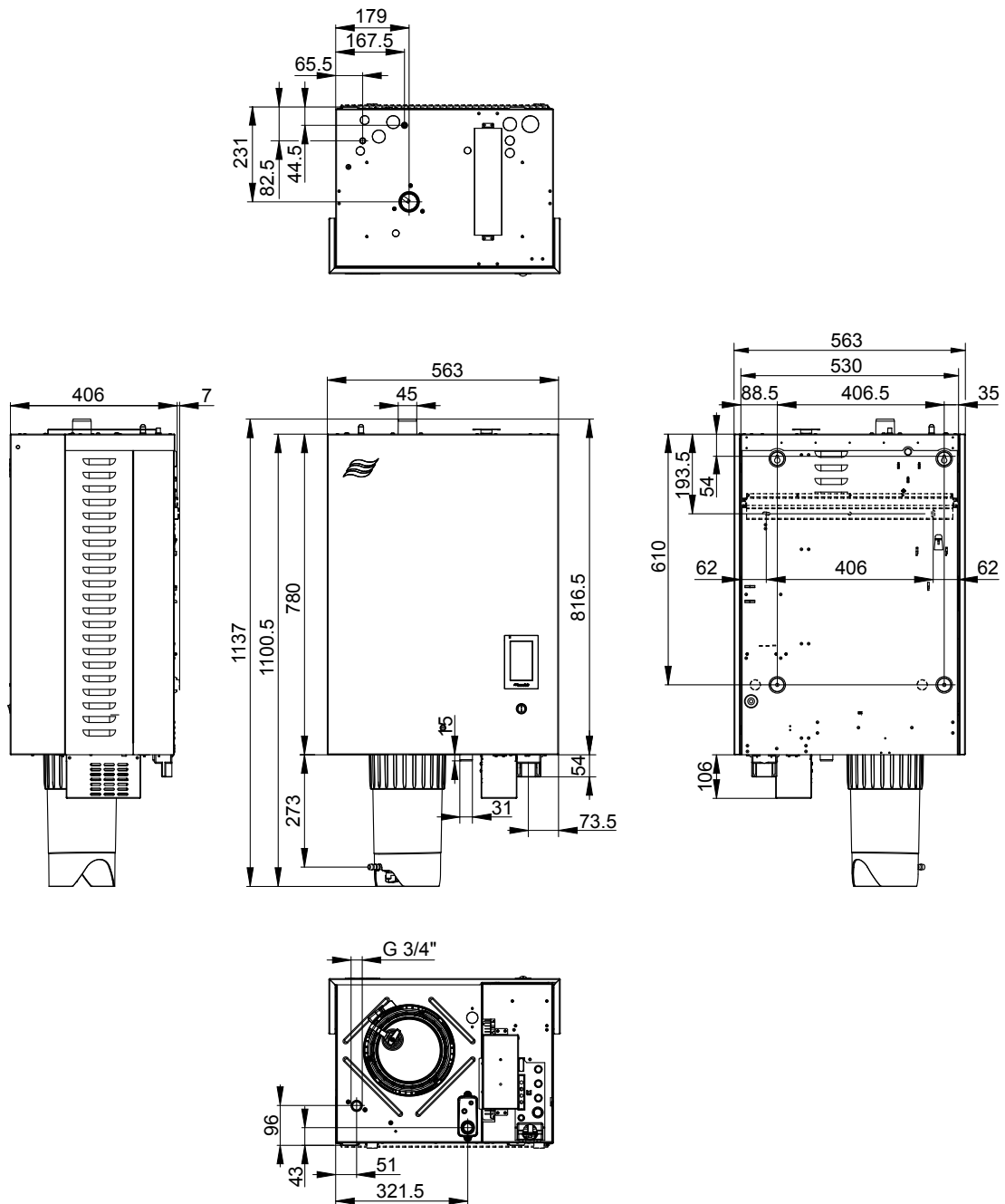
Fig. 35: Dimensioni del modulo "M" (misure in mm)
