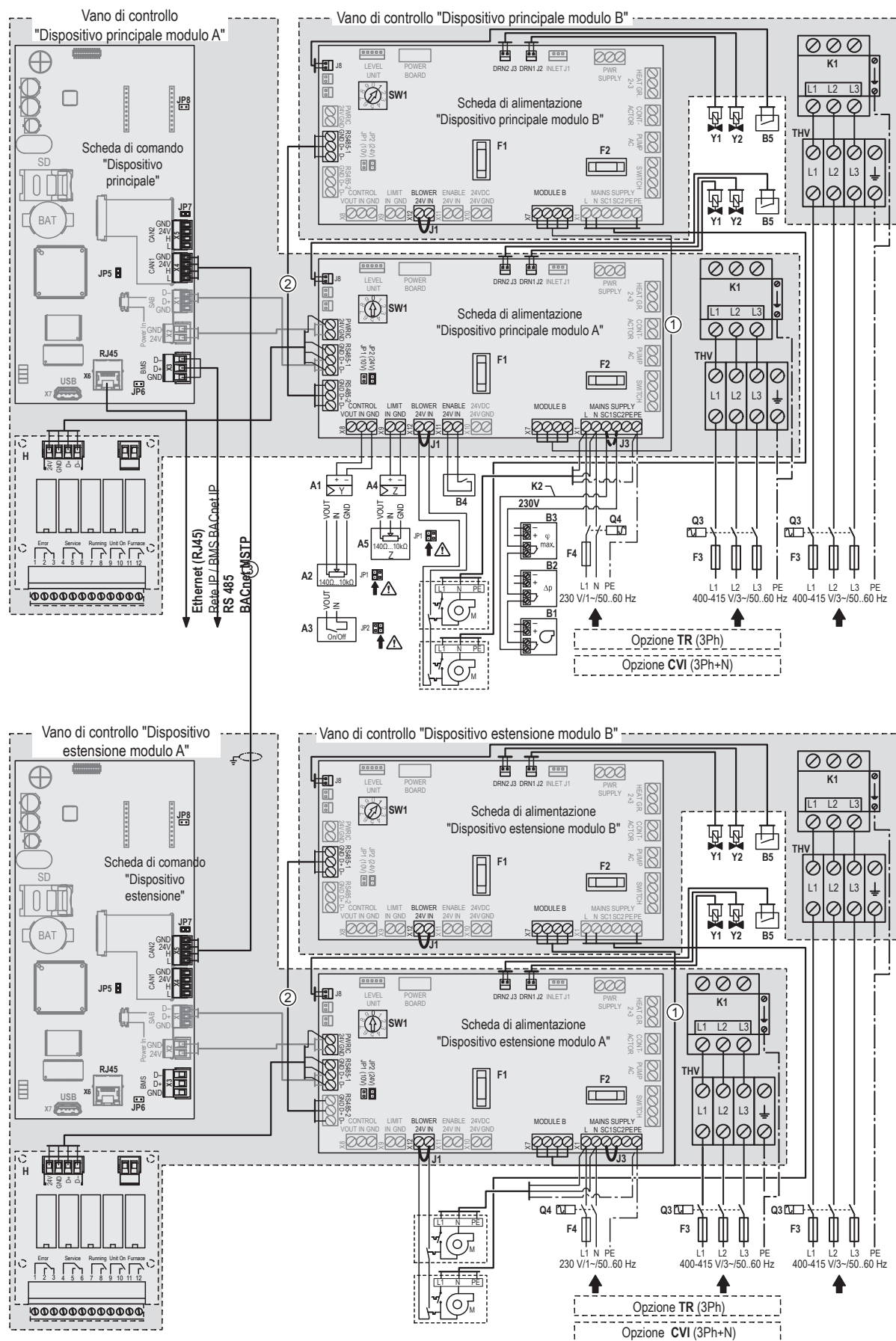
Fig. 31: Schema elettrico Condair RS - sistemi interconnessi (100...160 kg/h)
