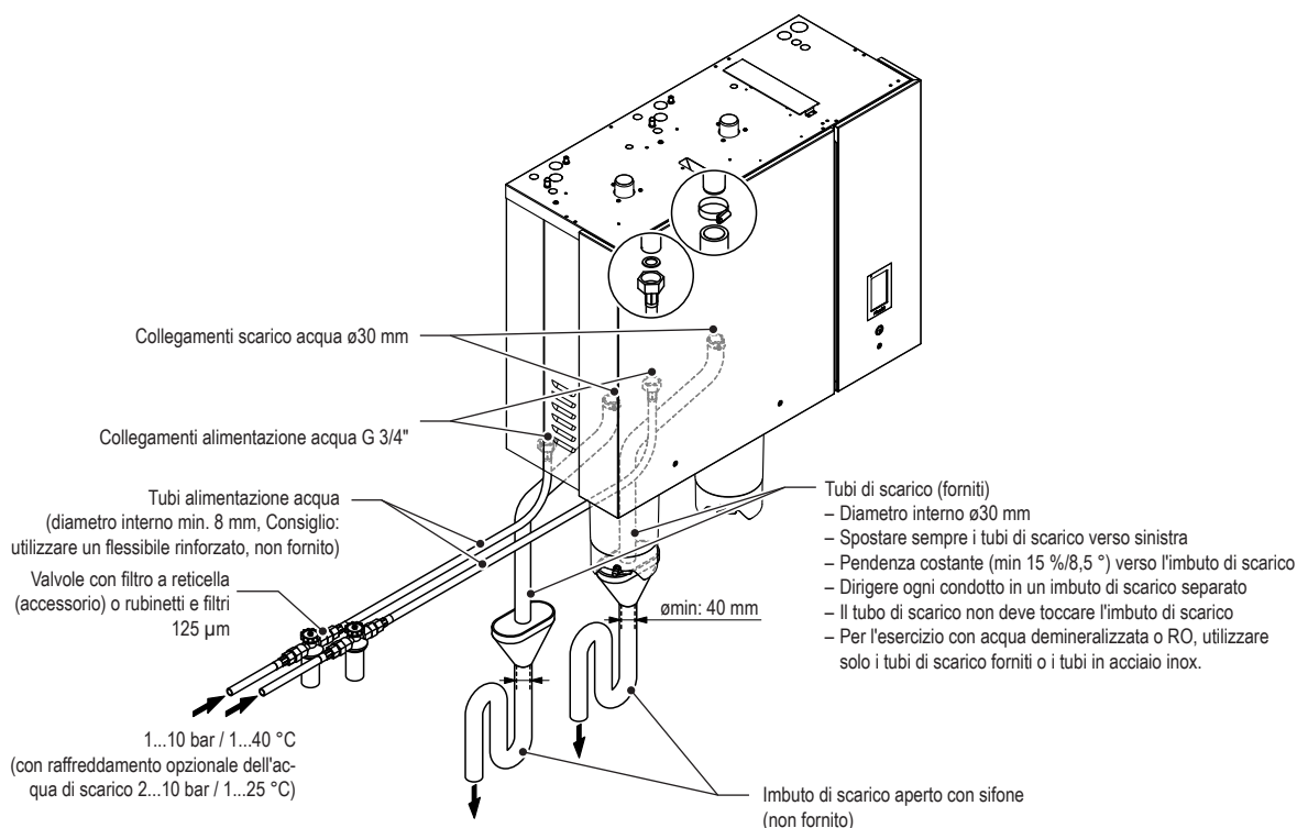
Fig. 23: Panoramica dell'installazione idraulica del singolo dispositivo grande
