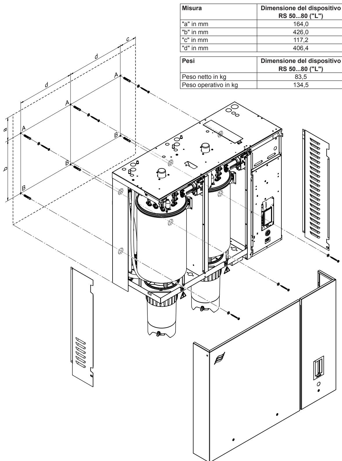
Fig. 12: Schema del montaggio standard dei moduli singoli grandi
