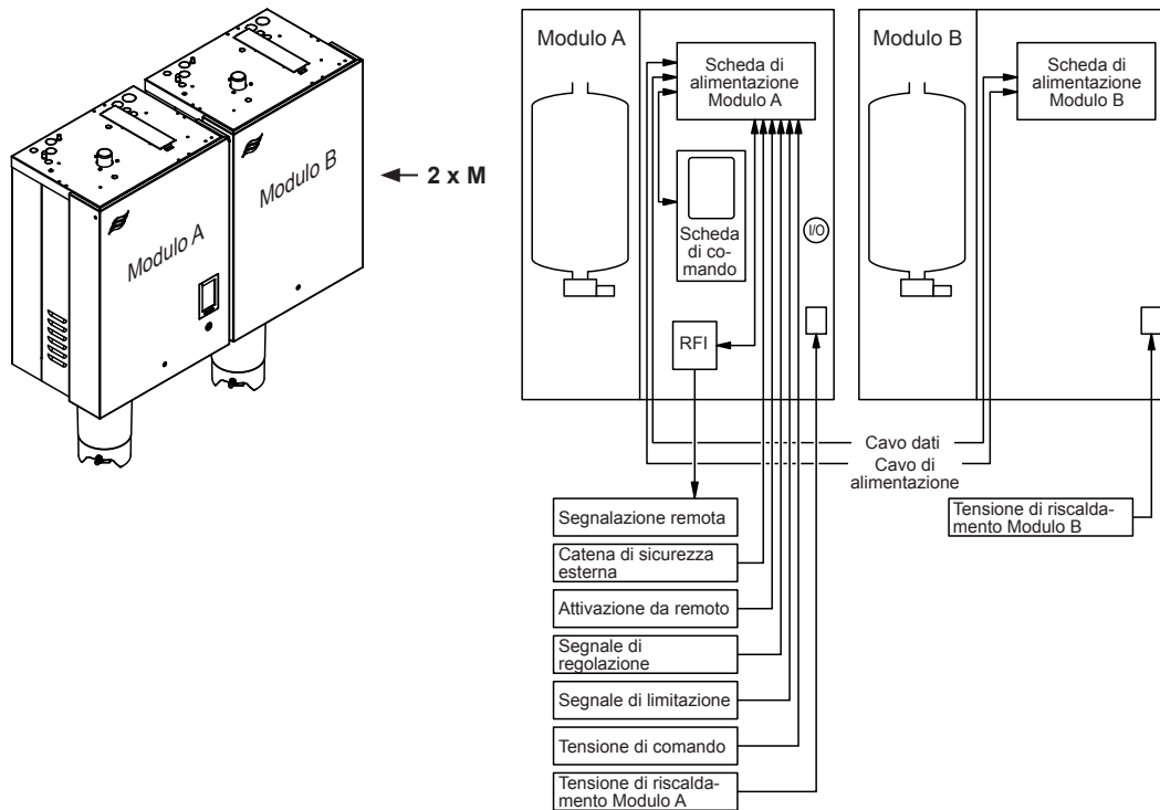
Fig. 3: Panoramica Moduli doppi (2 x "M")
