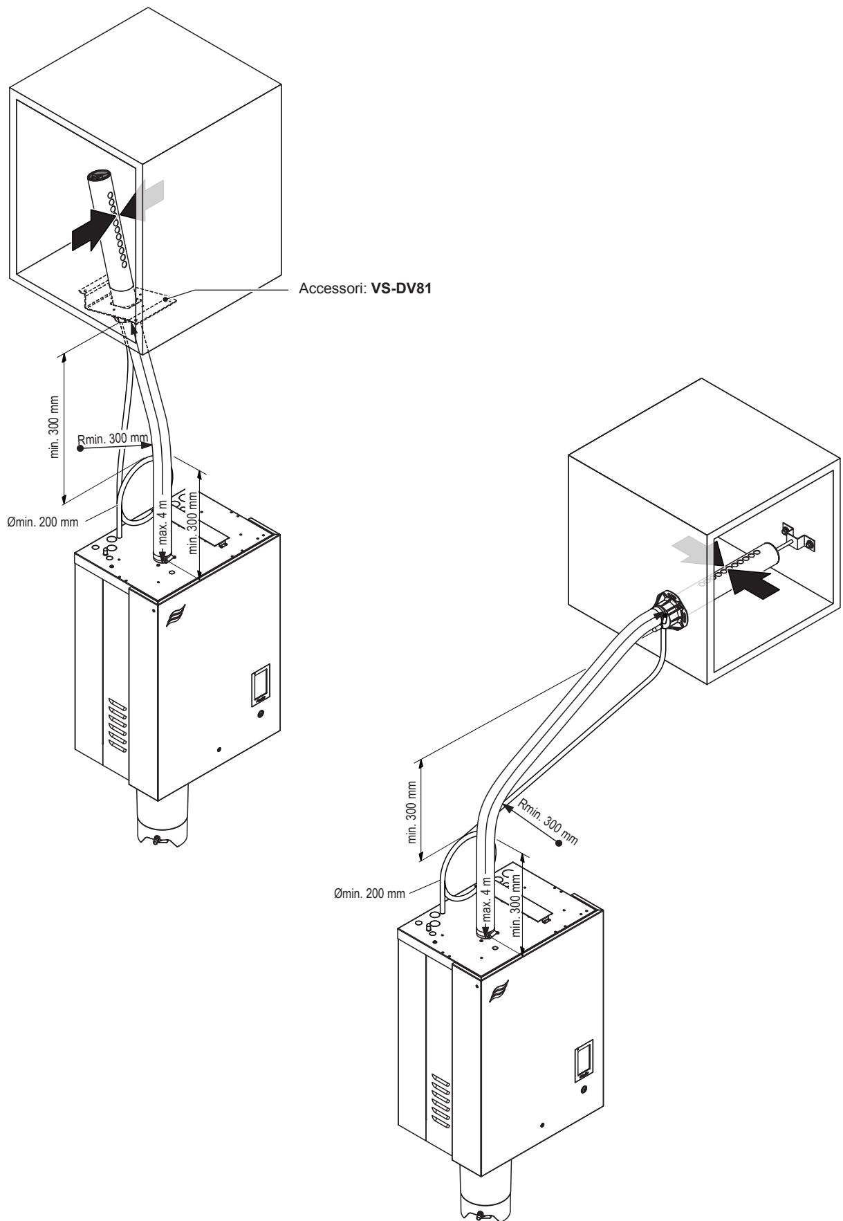
Fig. 18: Il distributore di vapore è montato a più di 500 mm sopra l'angolo superiore del dispositivo
