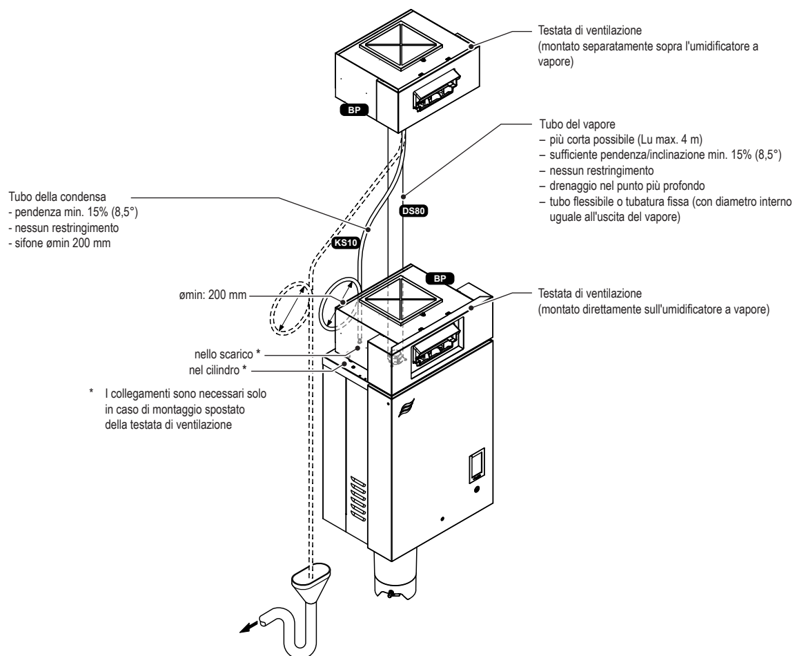
Fig. 16: Schema della distribuzione del vapore diretta in ambiente
