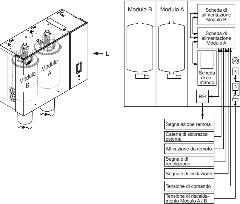
Fig. 2: Panoramica moduli singoli grandi ("L")
