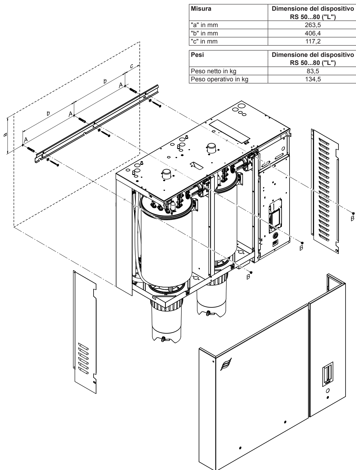
Fig. 14: Schema del montaggio dei moduli singoli grandi con barra di montaggio
