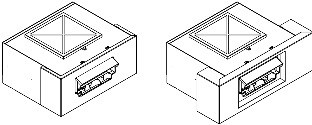
Fig. 7: Testata di ventilazione con pannello di copertura piccolo (a sinistra) e pannello di copertura grande (a destra)
