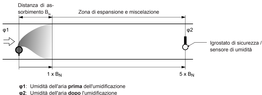
Fig. 17: Distanza di assorbimento "B N "
