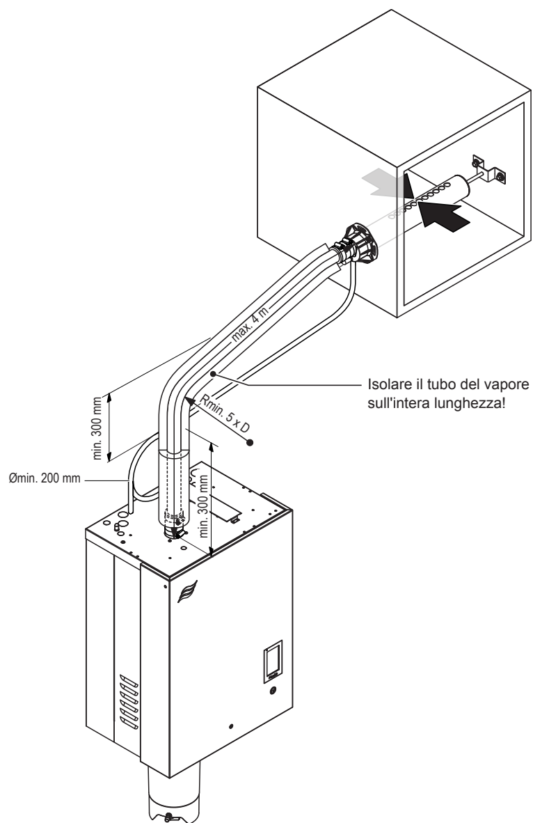
Fig. 20: Tubo del vapore con tubazioni fisse e isolamento
