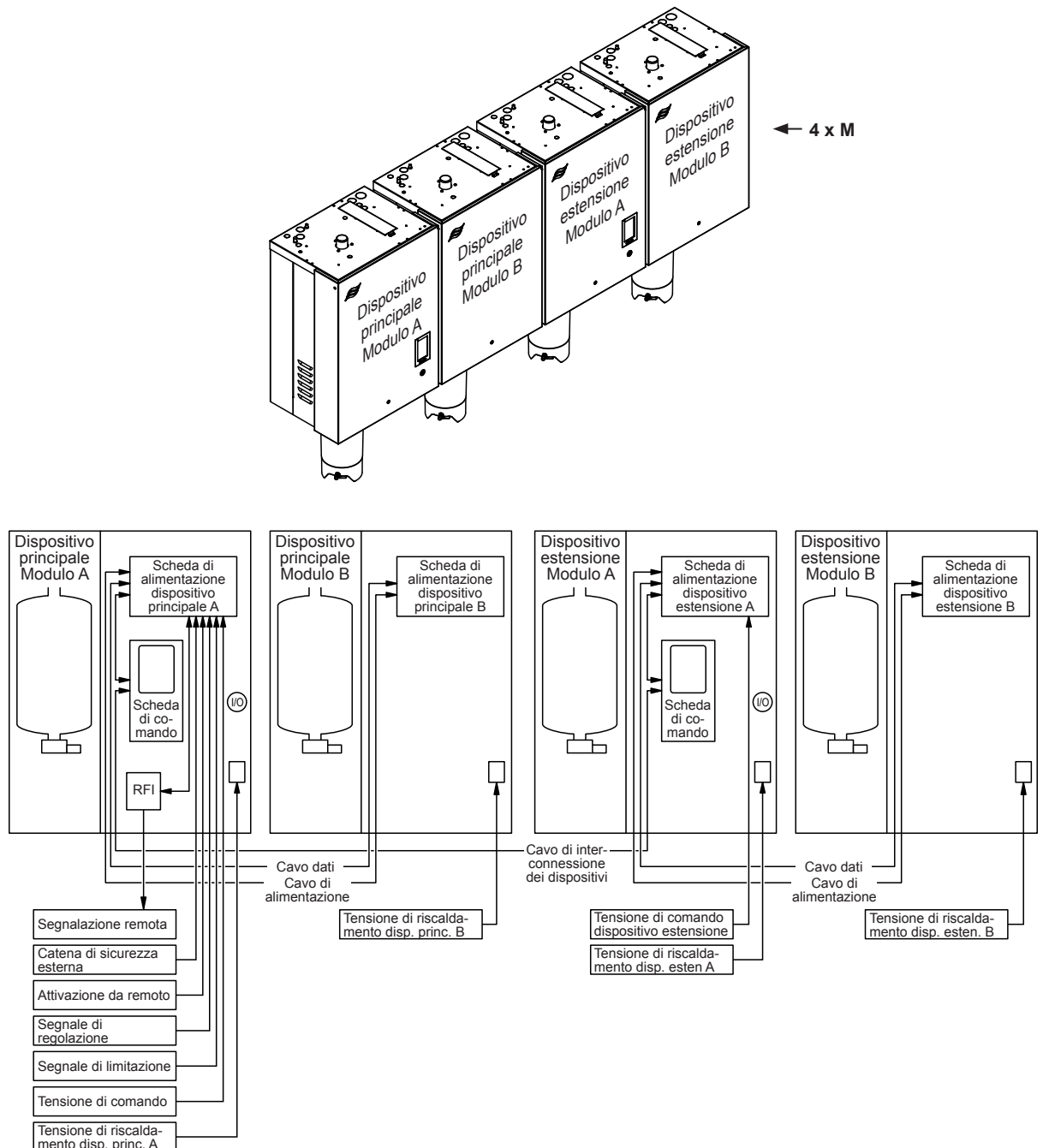
Fig. 5: Panoramica sistemi interconnessi (4 x "M")
