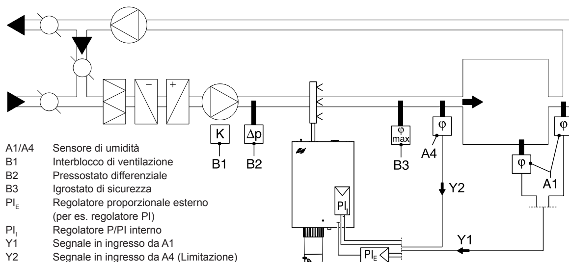
Fig. 26: Sistema 2 - Regolazione dell'umidità ambientale con limitazione proporzionale dell'umidità dell'aria di rinnovo
