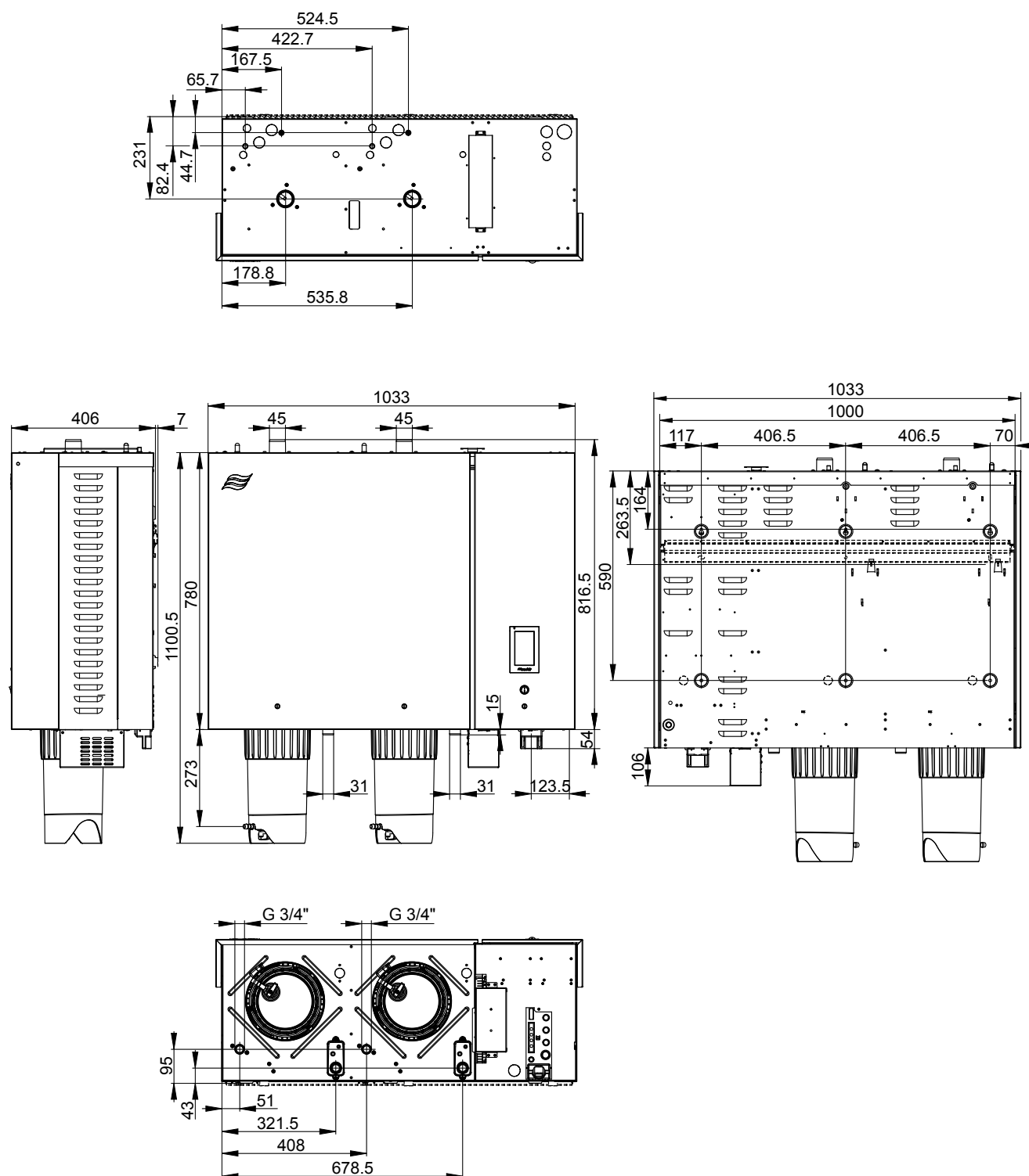
Fig. 36: Dimensioni del modulo "L" (misure in mm)
