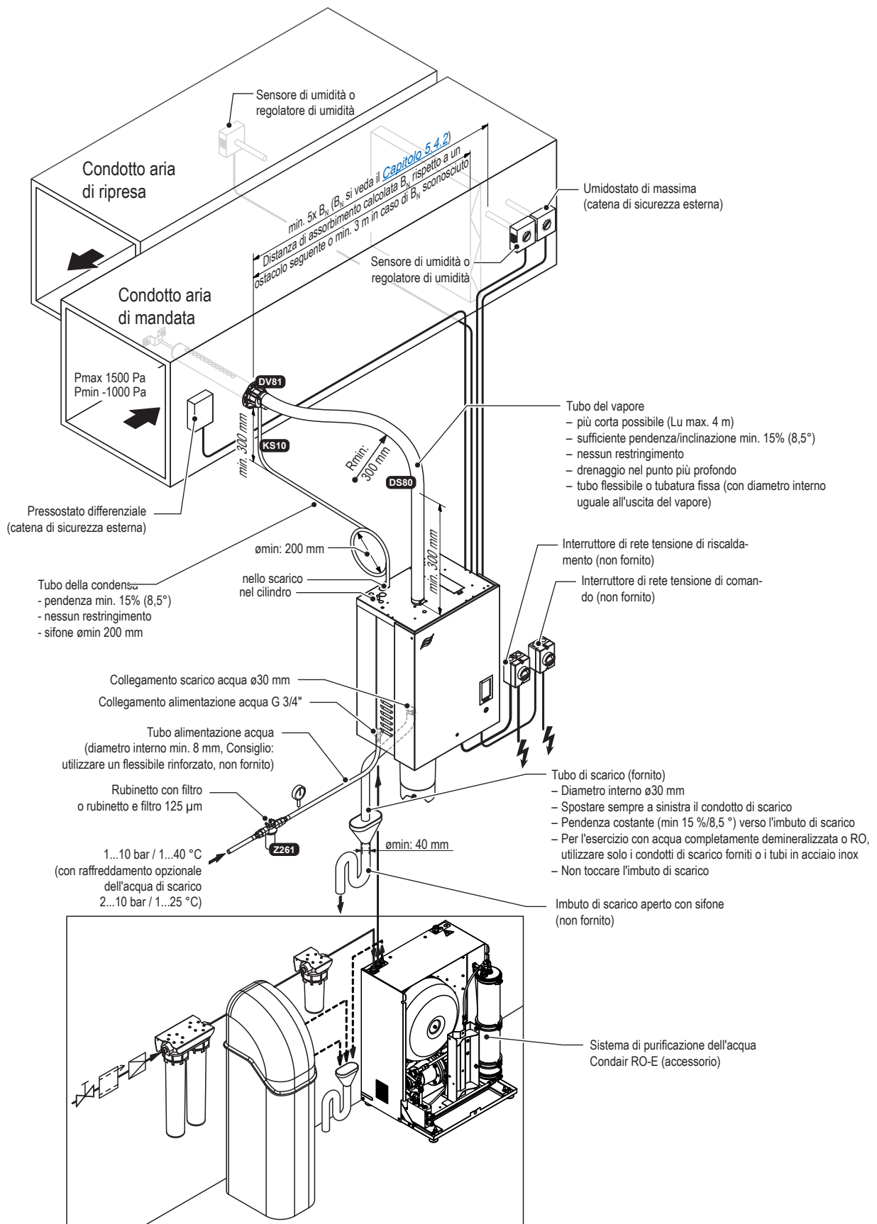
Fig. 8: Installazione tipica per l'umidificazione in canale
