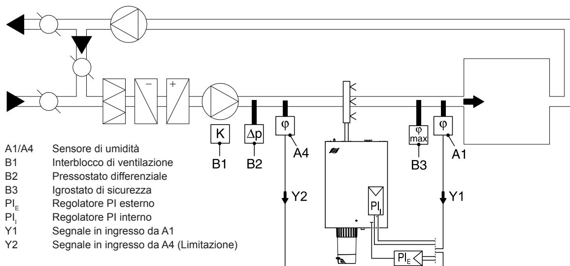
Fig. 27: Sistema 3 - Regolazione dell'umidità dell'aria di rinnovo con limitazione proporzionale dell'erogazione
