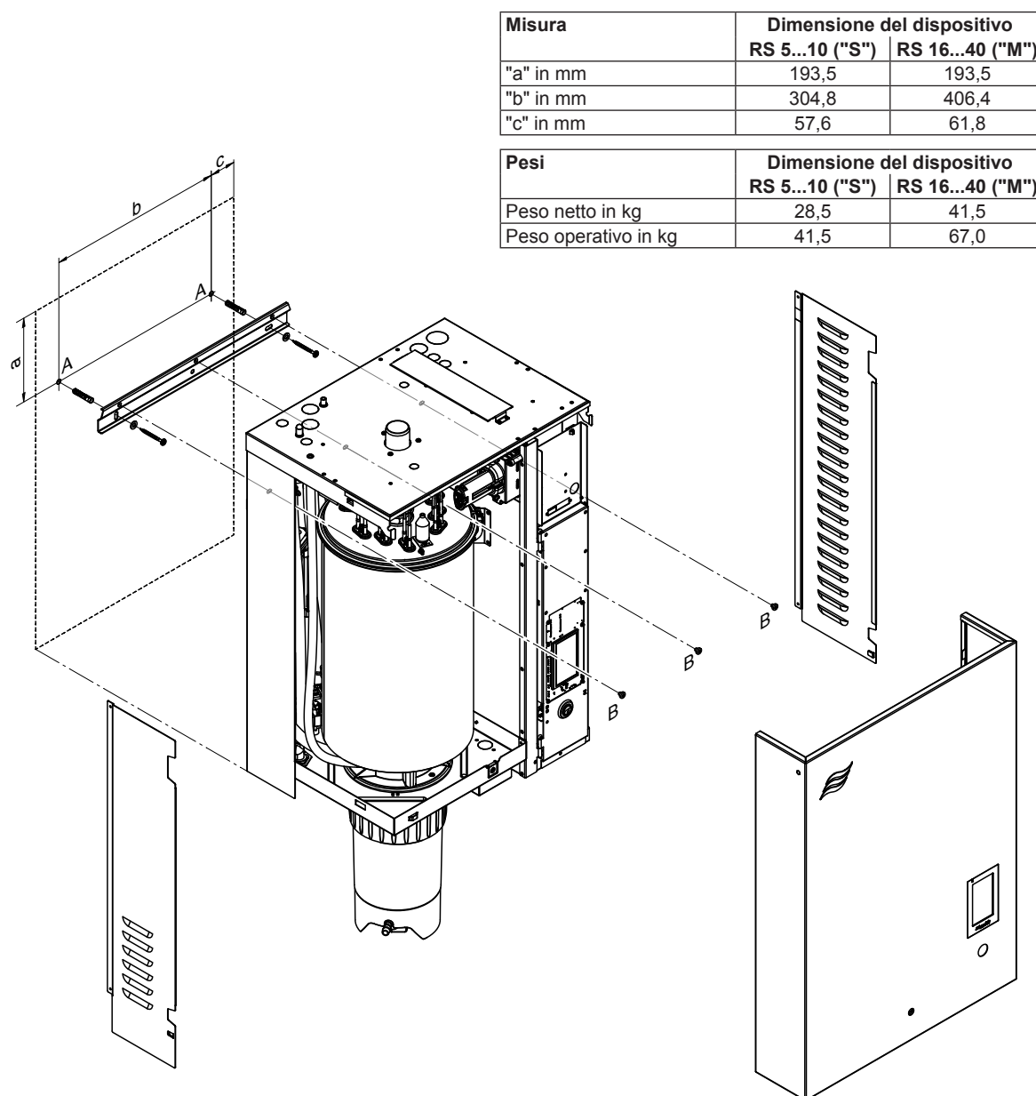
Fig. 13: Schema del montaggio dei moduli singoli piccolo e medio con barra di montaggio
