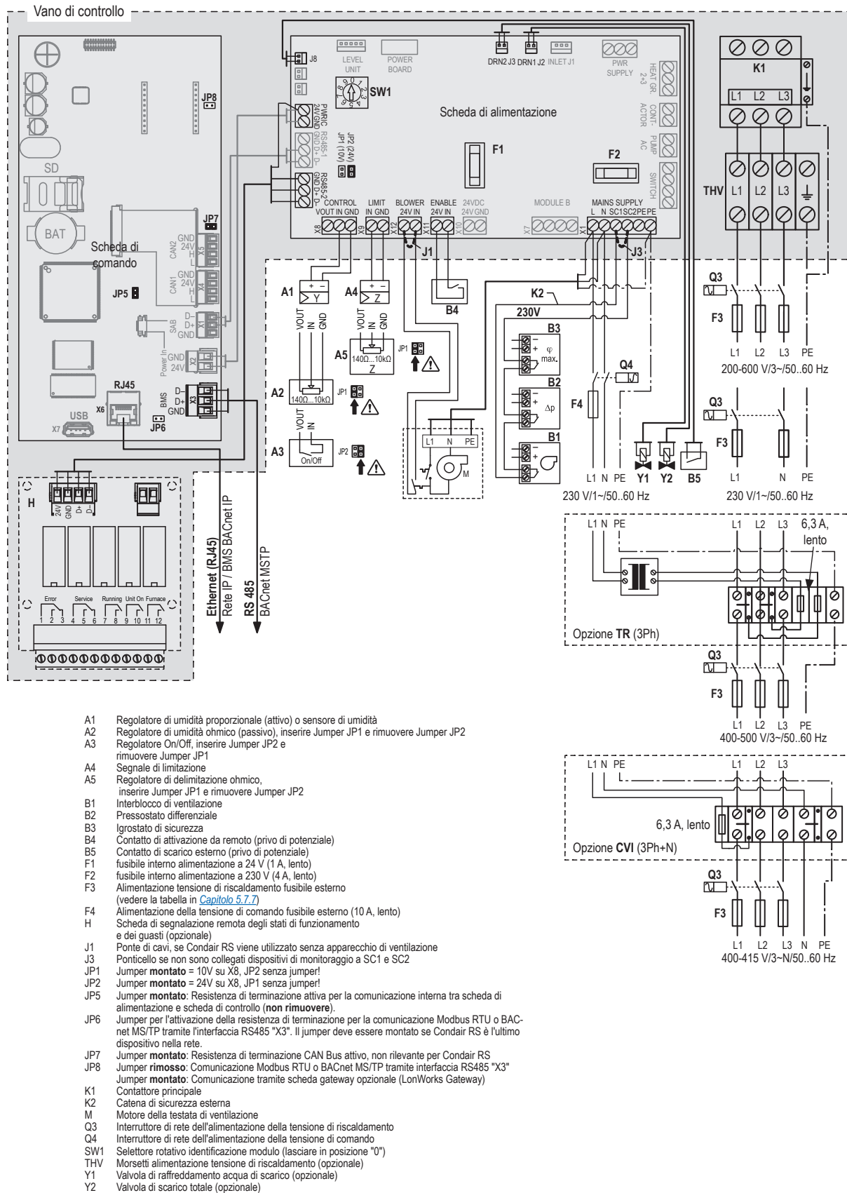
Fig. 28: Schema elettrico Condair RS - Moduli singoli piccolo "S" e medio "M" (5...40 kg/h)
