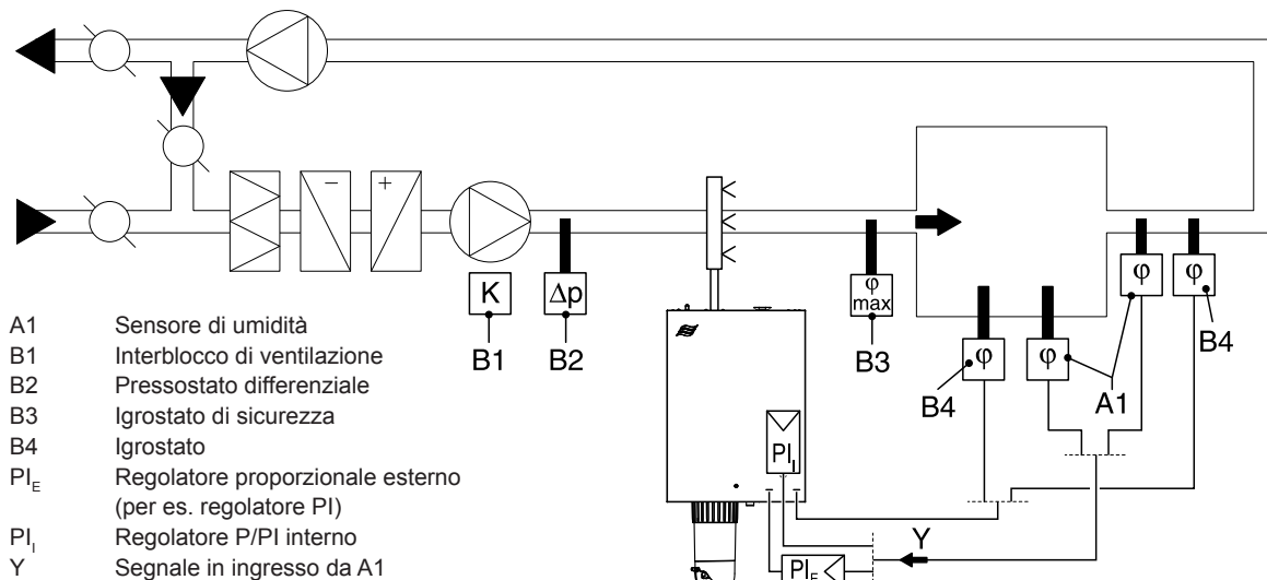
Fig. 25: Sistema 1 - Regolazione dell'umidità ambientale
