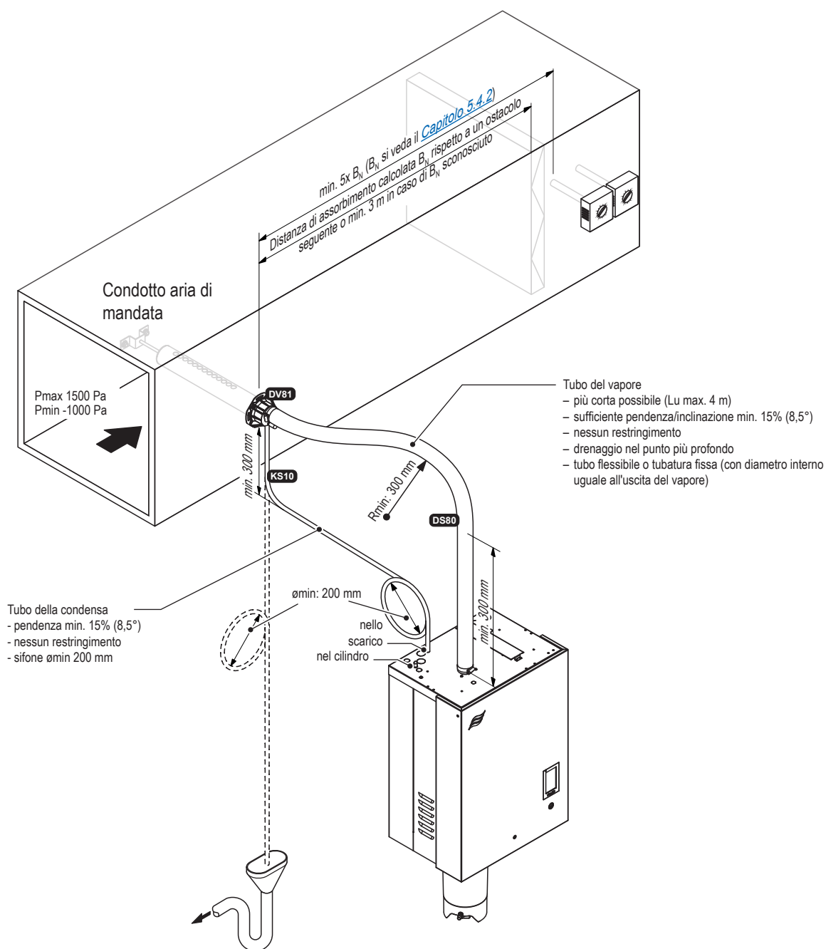
Fig. 15: Schema della distribuzione del vapore in canale
