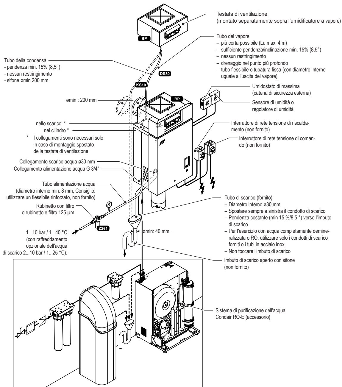
Fig. 9: Installazione tipica per l'umidificazione diretta in ambiente
