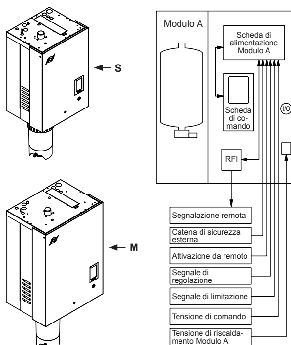
Fig. 1: Panoramica moduli singoli piccolo ("S") e medio ("M")
