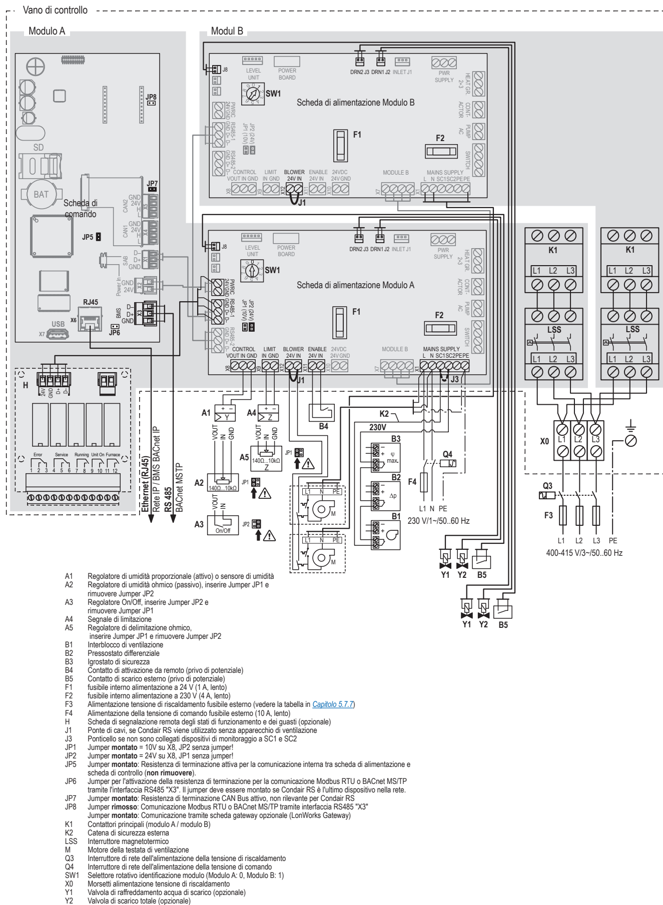
Fig. 29: Schema elettrico Condair RS - Moduli singoli grande "L" (50...80 kg/h)
